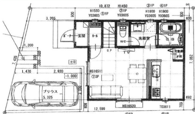
1階平面図
